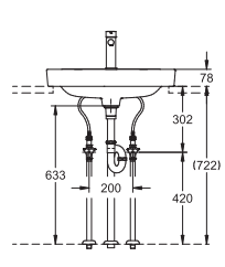
床給水・床排水仕様 参考図
