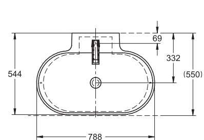
ユーロコスモ ベッセル洗面器 39070 タイプ
