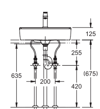
床給水・床排水仕様 参考図
