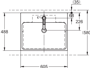
スクエア型 オーバーカウンター洗面器 39311 タイプ
