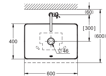
ユーロセラミック ベッセル洗面器 10243 タイプ
