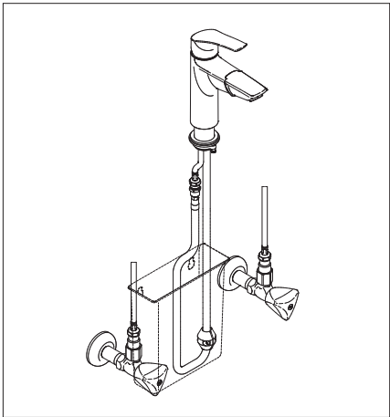
【水受容器設置例】 キッチン水栓
