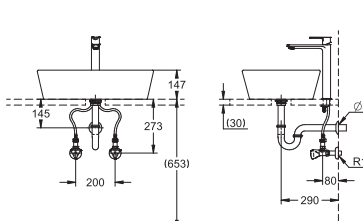
壁給水・壁排水仕様 参考図
