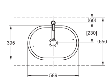
ユーロコスモ ベッセル洗面器 39122 タイプ
