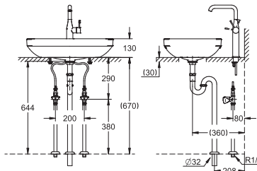
床給水・床排水仕様 参考図
