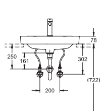
壁給水・壁排水仕様 参考図
