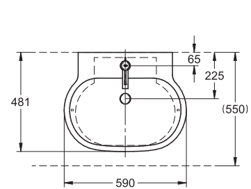
ユーロコスモ ベッセル洗面器 39291 タイプ
