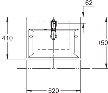
スクエア型ベッセル洗面器 JPK102 タイプ
