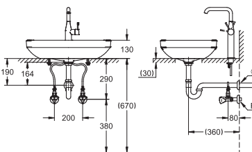
壁給水・壁排水仕様 参考図
