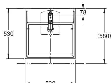
スクエア型ベッセル洗面器 JPK111 タイプ
