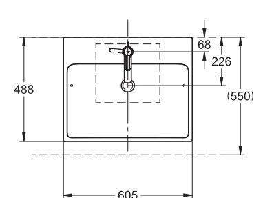
ユーロキューブ ベッセル洗面器 39234 タイプ
