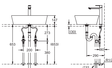
床給水・床排水仕様 参考図
