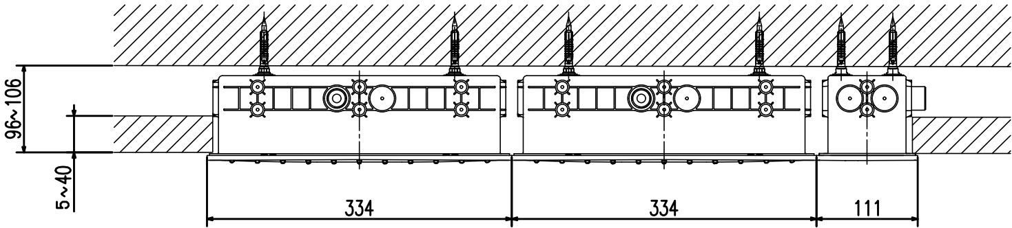
＜天井設置イメージ＞
