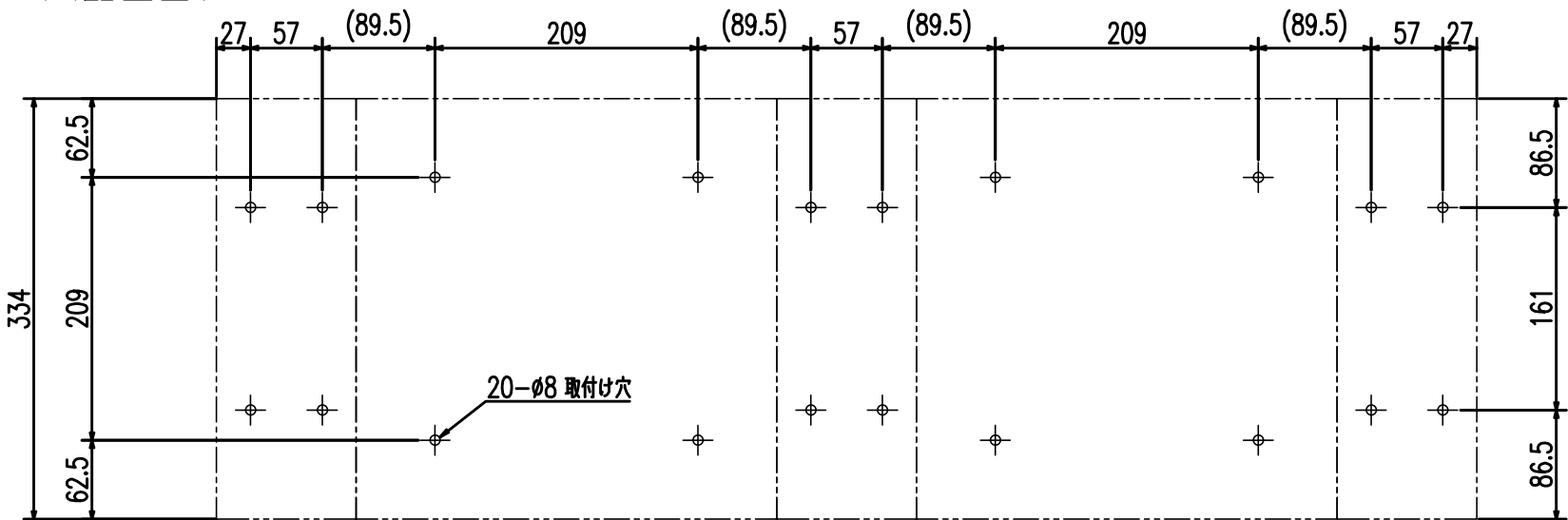
＜取付け穴配置図＞
