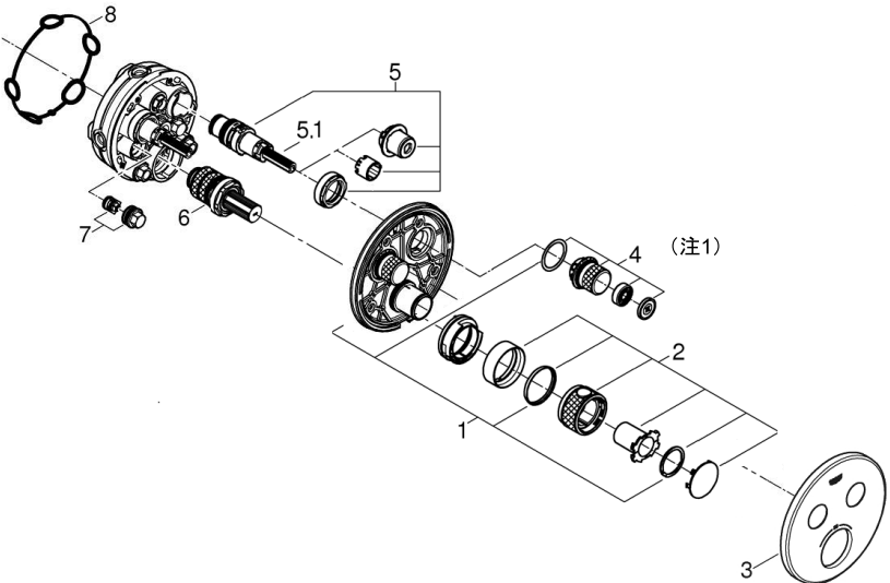
5.1 : 高さ調整ねじ部分のみ
