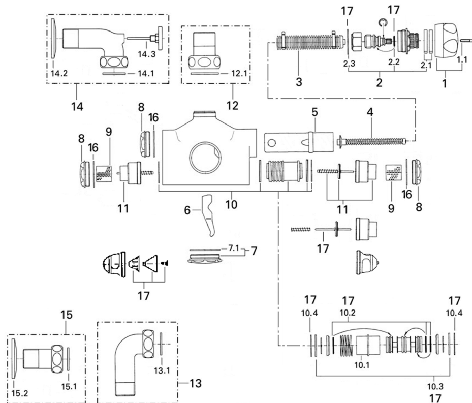
図番17: 47029000 「35089・35121修理用Oリングセット」 セット内容
