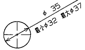
カウンター穴寸法
