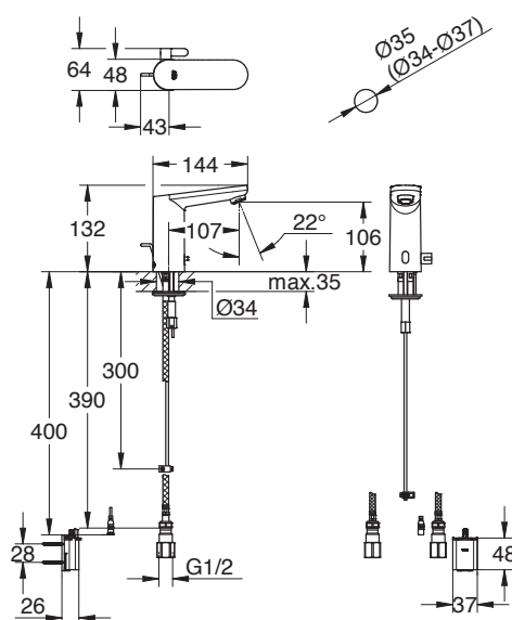
自動混合栓(引棒付) JP 2109 00 ¥65,000 クローム
